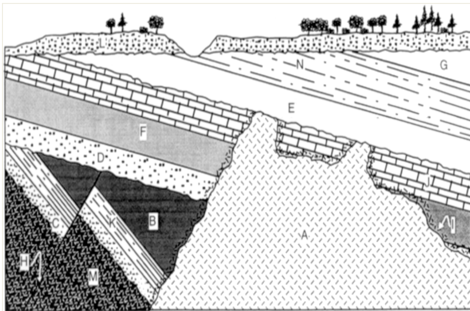
Coupe géologique N°3 ( ne pas tenir compte de l'évènement géologique I )
