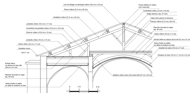
Coupe transversale de charpente
