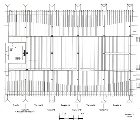
Plan de charpente
